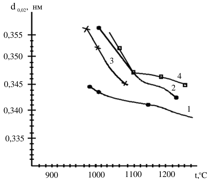
Рисунок 3.6 - Зависимость изменения межплоскостного расстояния d_{002} антрацитов от температуры термообработки: 1. - антрацит российского Донбасса (ш. им. 60-летия Ленинского комсомола); 2- антрацит Донецкого бассейна 3.- антрацит месторождения Назарайлок участок «Шикорхона» 4.- антрацит Горловского бассейна (Россия)
