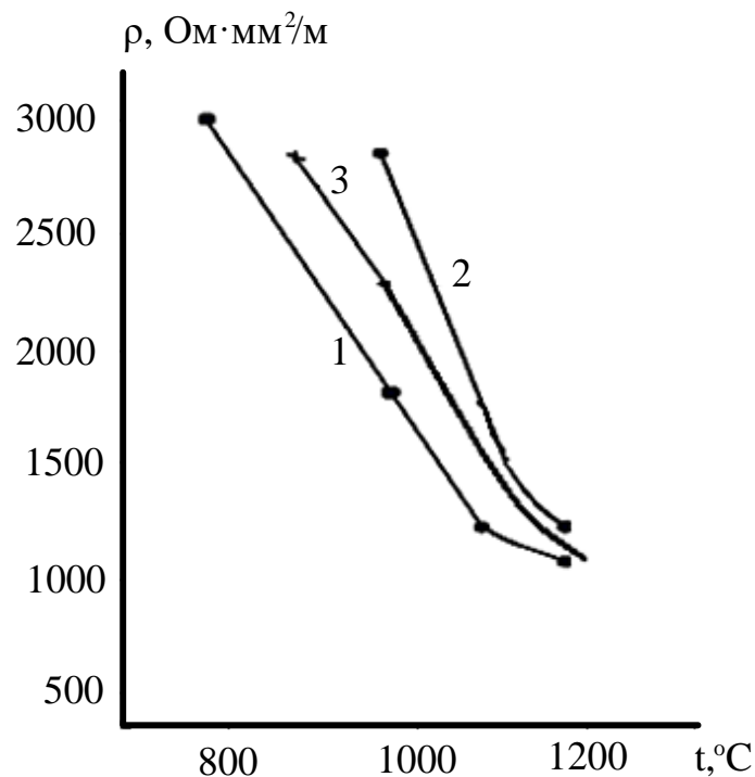
Рисунок 3.3 - Изменение удельного электросопротивления антрацитов в зависимости от температуры обработки: 1 – Донецкий бассейн; 2–Горловский бассейн; 3 – Назарайлокский антрацит
