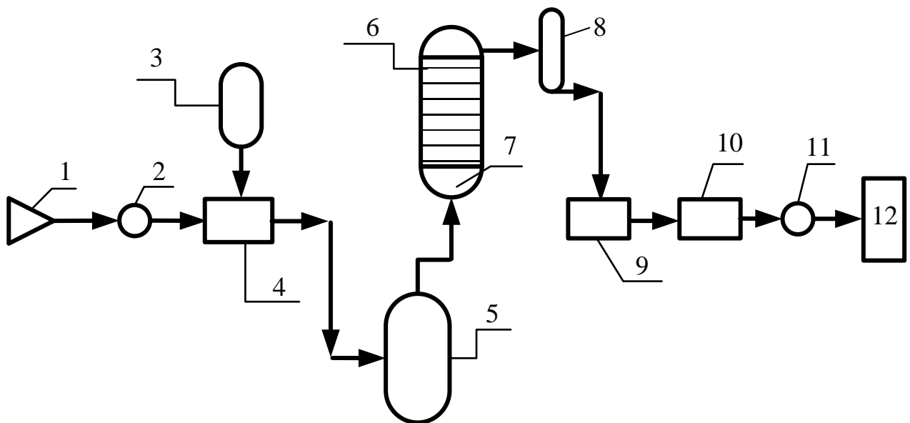
Рисунок 5.1. Схема лабораторной установки по газификации угля: 1-компрессор; 2-расходомер; 3-резервуар для воды; 4-гидрозатвор; 5-парообразователь с пароперегревателем; 6-реактор (газогенератор (ГГ)); 7-электронагреватель для ГГ; 8-холодильник; 9-сепаратор; 10-фильтр; 11-газовый счетчик; 12-блок анализа
