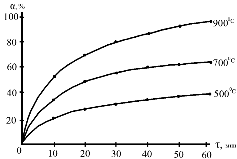
Рисунок 2.5 - Зависимость степени выхода смеси газов от продолжительности прокалики антрацита при разных температурах
