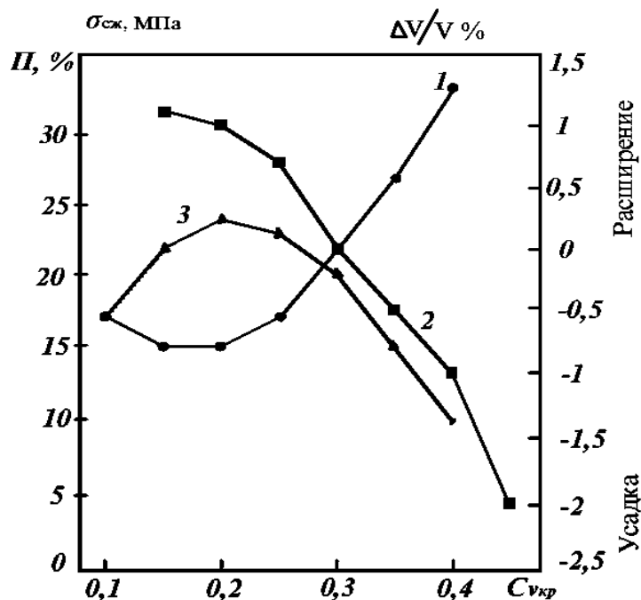
Рисунок 3.1 - Влияние объемной доли крупной фракции C_{вкр} на пористость \Pi (1), объемные изменения (2) и механическую прочность при сжатии (3) при условии постоянной внешней удельной поверхности шихты
