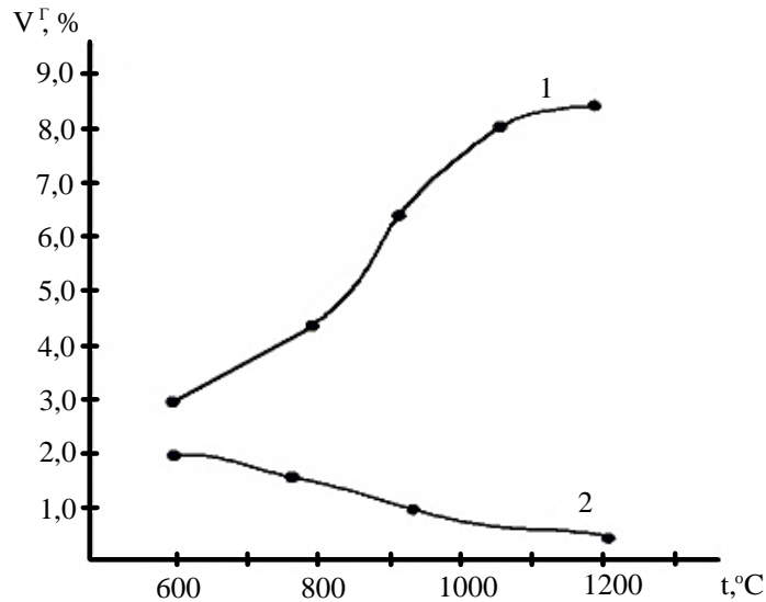
Рисунок 3.4 - Зависимость выхода летучих от температуры прокалки:
