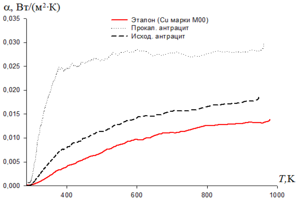
Рисунок 2.16 - Температурная зависимость коэффициента теплоотдачи эталона и антрацитов
