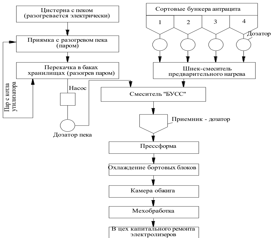
Рисунок 4.6 -Принципиальная технологическая схема производства бортовых блоков ОАО «ТАЛКО»
