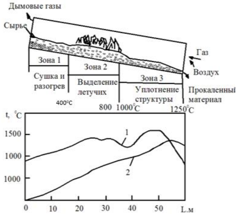
Рисунок 3.15 - Схематическая диаграмма зон прокаливания углеродного сырья и температурные профили газového потока 1 и слоя материала 2 по длине печи
