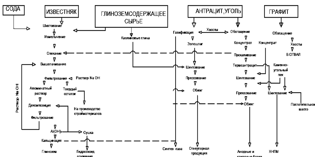
Рисунок 5.4 - Принципиальная технологическая схема комплексной переработки углеродсодержащего минерального сырья
