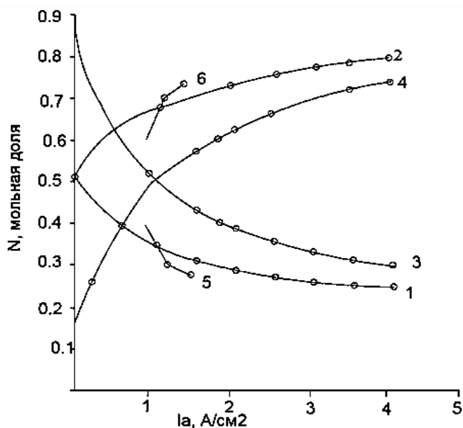
Рисунок 4.8 - Зависимость мольных долей CO(1,3,5) и CO 2 (2,4,6) от анодной плотности тока ( T=1233 K): 1,2 – стандартные аноды; 3,4 – нестандартные аноды; 5,6 – данные [192, 198-202]
