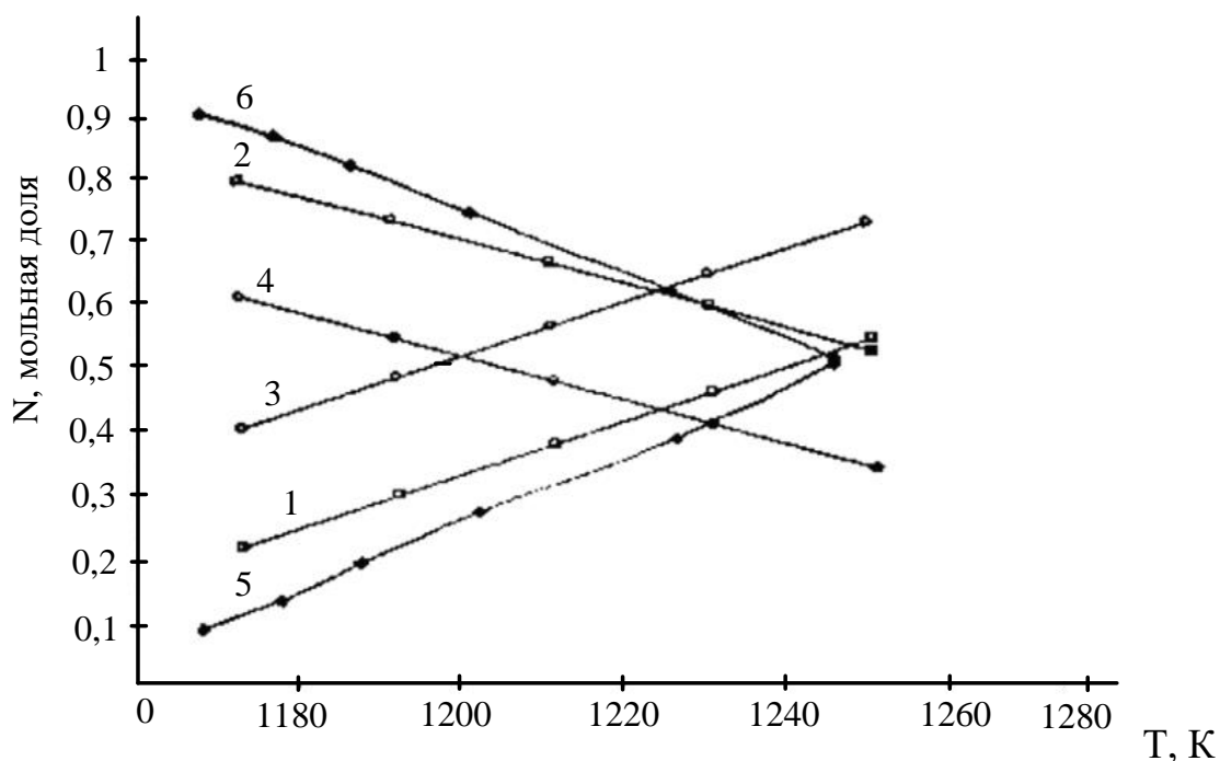
Рисунок 4.9 - Зависимость мольных долей CO (1,3,5) и CO 2 (2,4,6) от температуры ( i_a=0.8 A/cm 2 ): 1,2 – стандартные аноды; 3,4 – нестандартные аноды; 5,6 – данные [199]
