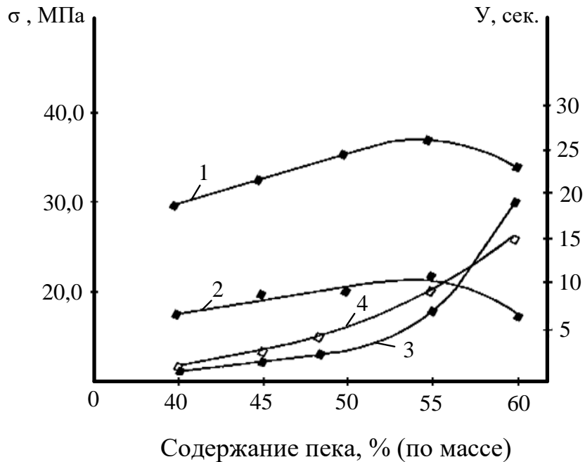
Рисунок 3.9 - Зависимость механической прочности ( \sigma ), уплотняемости ( У ) ХНПМ от содержания пека в связующем: 1 – \sigma (Назарайлок); 2 – \sigma (Запорожье); 3- У (Запорожье); 4- У (Назарайлок)
