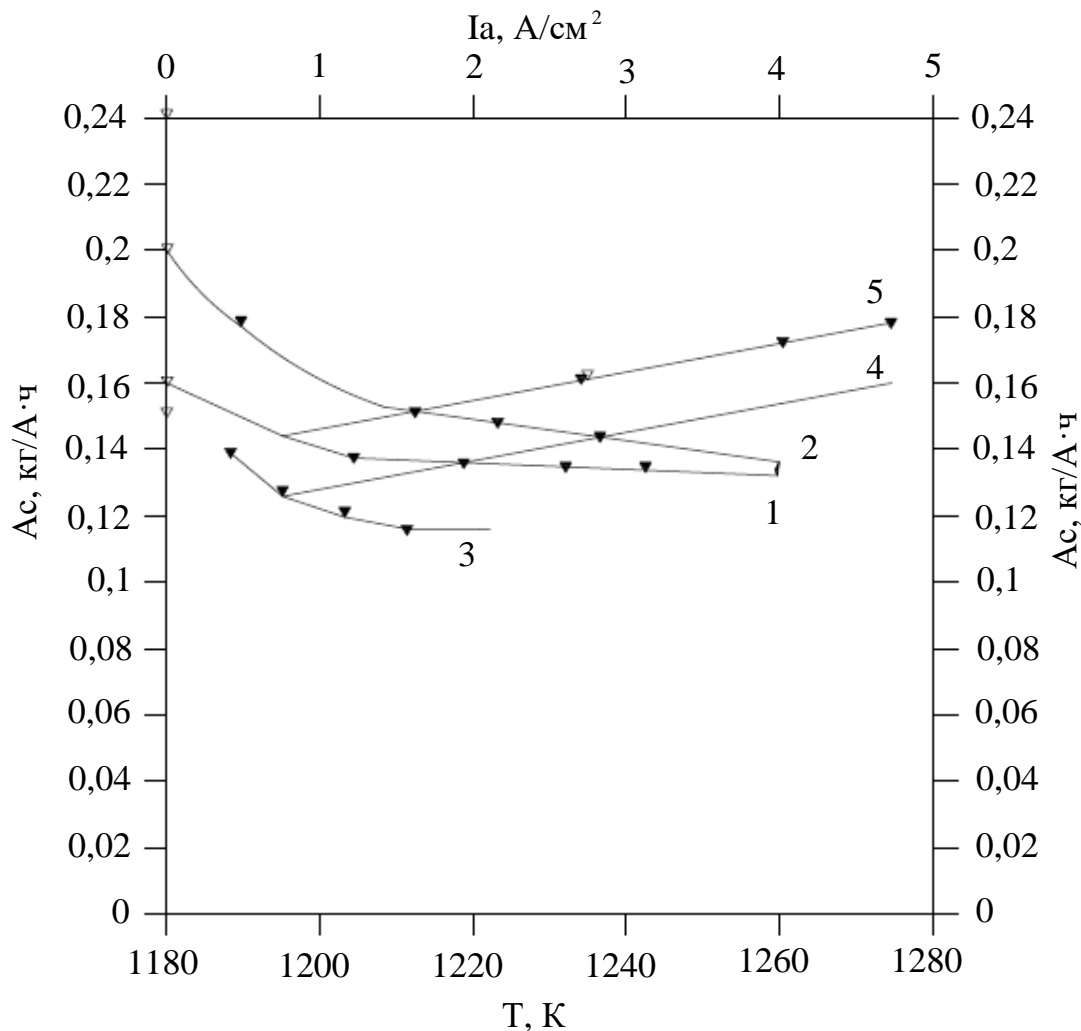
Рисунок 4.10 - Зависимость удельного расхода углерода от плотности тока (1,2,3) и температуры (4,5): 1,4 - стандартные аноды; 2,5 - нестандартные аноды; 3- данные [192]
