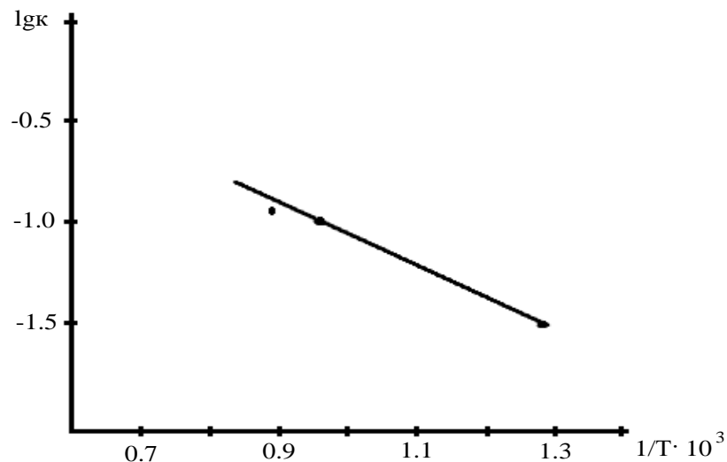
Рисунок 2.7 - Зависимость \lg K от величины обратной температуры
