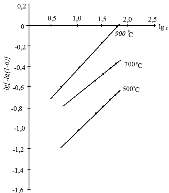
Рисунок 2.6 - Зависимость \lg[-\lg(1-\alpha)] от \lg t при разных температурах
