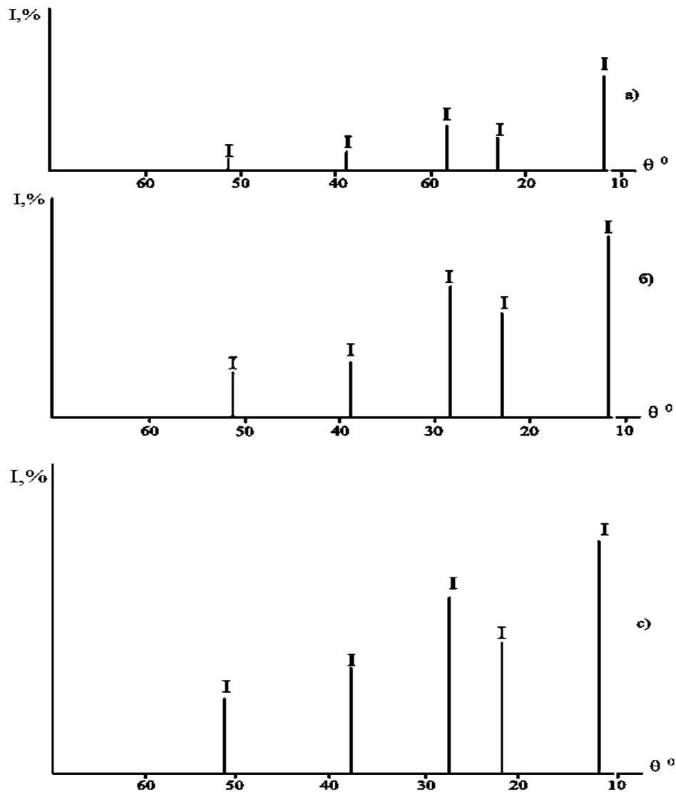
Рисунок 2.8 - Штрихрентгенограммы: а) исходный антрацит; б) антрацит после прокалики (при температуре 1200^{\circ}\text{C} ); антрацит после прокалики (при температуре 1400^{\circ}\text{C} )
