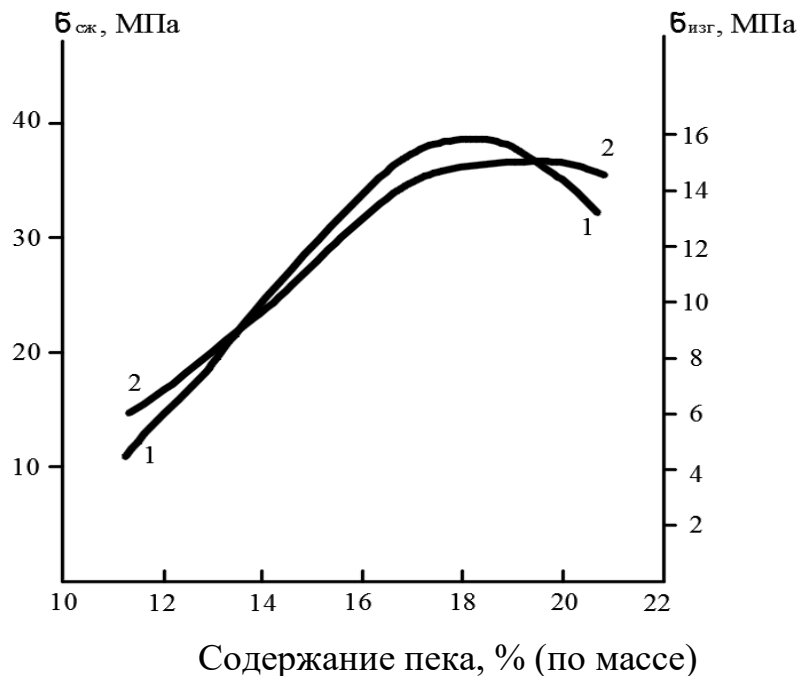
Рисунок 4.3 - Зависимость предела прочности на сжатие ( b_{сж} ) и предела прочности на изгиб ( b_{изг} ) от количества связующего (пека): 1- предел прочности на сжатие; 2- предел прочности на изгиб
