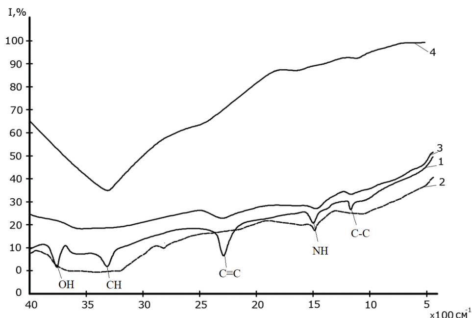
Рисунок 2.12 - ИК-спектры сырого и термообработанного антрацита месторождения Назарайлок (пласт №4): 1- сырой антрацит; 2 - термообработанный при 1000 0 С; 3- термообработанный при 1200 0 С; 4 - термообработанный при 1400 0 С
