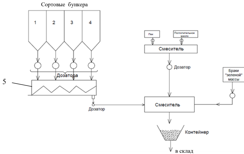
Рисунок 1.3 - Принципиальная технологическая схема производства ХНПМ. 1,2,3,4- сортовые бункера с разными фракциями, 5- шнек предварительного смешивания
